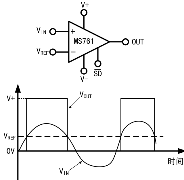
图1 简单比较器
